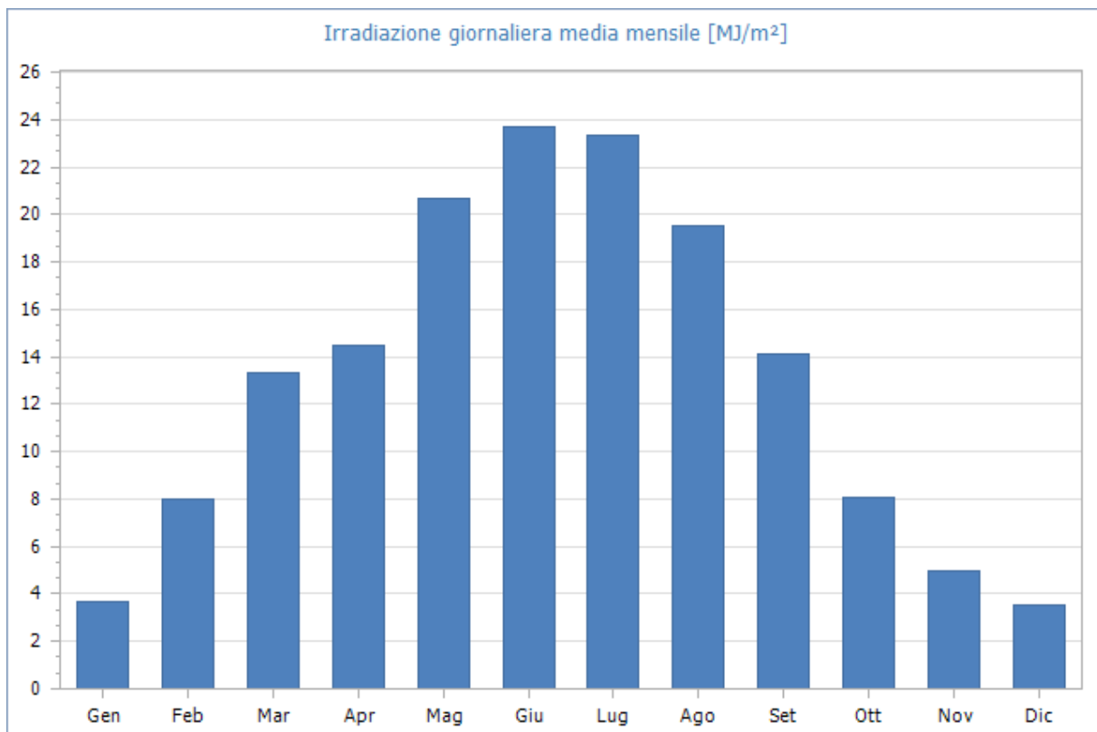
Fig. 1: Irradiazione giornaliera media mensile sul piano orizzontale [MJ/m 2 ]- Fonte dati: UNI 10349:2016 - Stazione di rilevazione: Castello di Agogna
